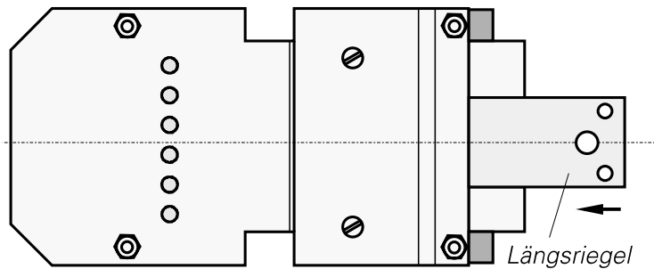
Standardausführung (Längsriegelplatte)
